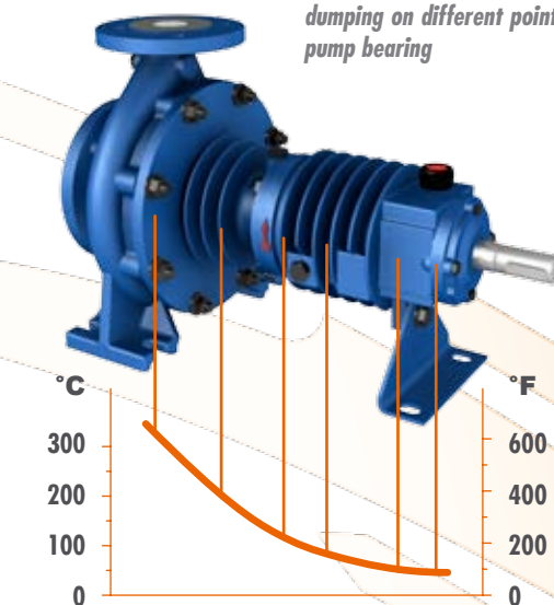
Diagramma dimostrativo dell'abbattimento del calore nei vari punti della supportazione
