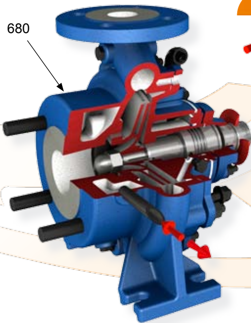
Esecuzione con corpo pompa e camera tenuta meccanica riscaldati o raffreddati (costruzione .../1X-R/.../T-U2) Construction with heated or cooled pump casing and mechanical seal chamber (design .../1X-R/.../T-U2)
