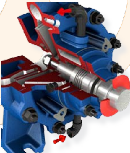
Esecuzione con corpo pompa e camera tenuta meccanica riscaldati o raffreddati (costruzione .../1X-R/.../T-U2) Construction with heated or cooled pump casing and mechanical seal chamber (design .../1X-R/.../T-U2)
